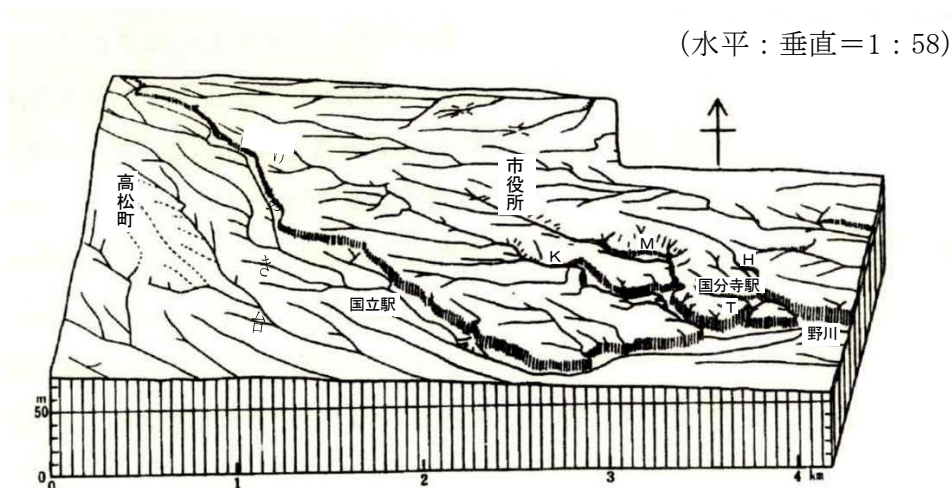
図1-3：国分寺市の地形ブロックダイアグラム
