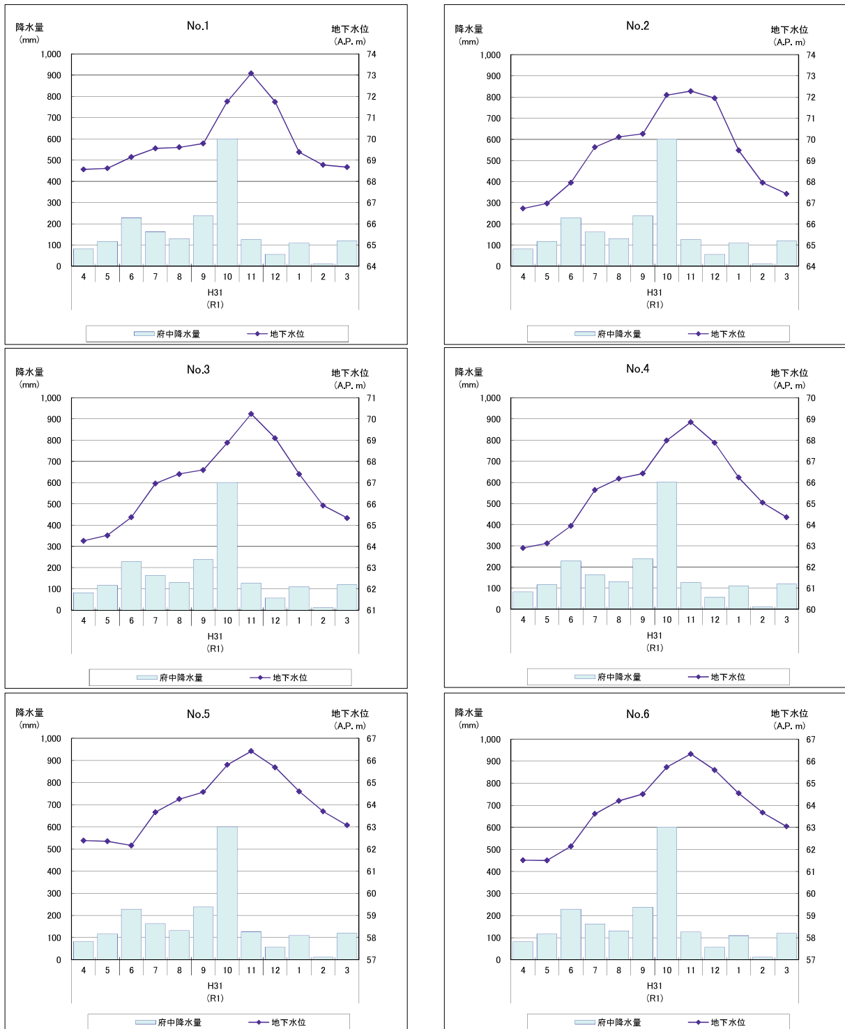
図-3.2(1) 地下水位測定結果及び気象庁府中観測所雨量 (1/6)
