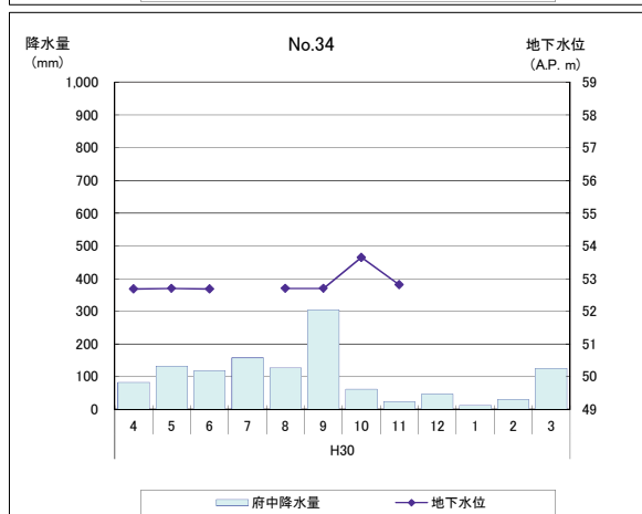
図-3.2(5) 地下水位測定結果及び気象庁府中観測所雨量 (5/6)
