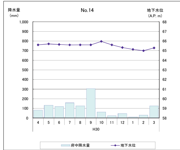
図-3.2(2) 地下水位測定結果及び気象庁府中観測所雨量 (2/6)
