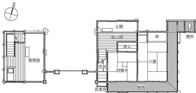
1階平面図
