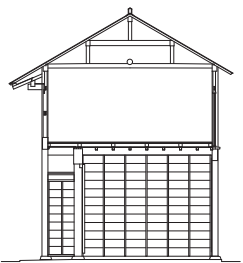
梁間断面図
