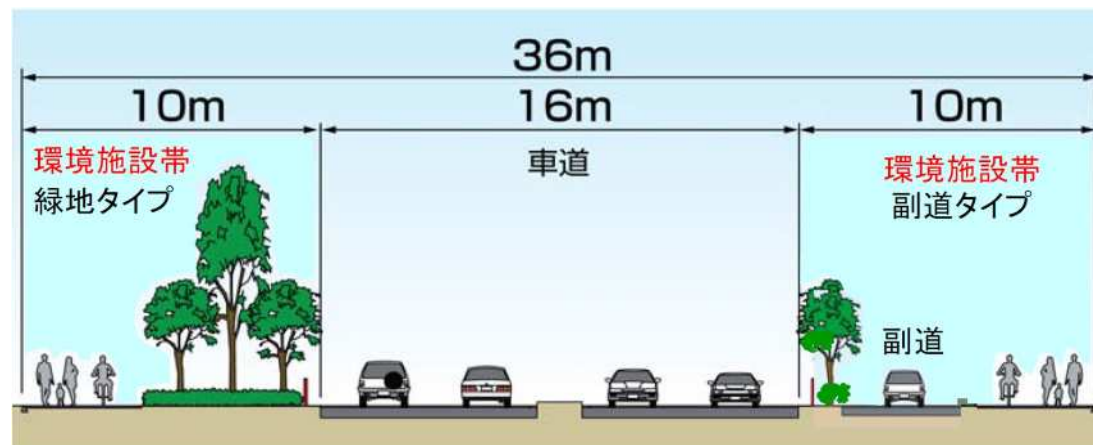
横断面図（イメージ図）
