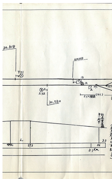
図 21 国分寺付近路線図
