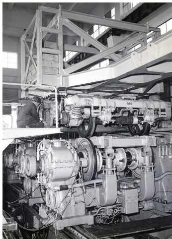
図 30 新幹線用高速台車試験 1960 年代 鉄道博物館所蔵
